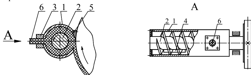
Рис. 2.3. Шнековое отборочное устройство:
