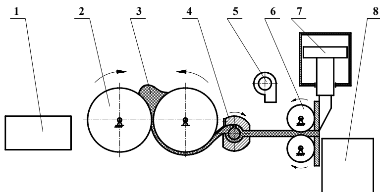
Рис. 2.1. Технологический процесс вторичной переработки отходов термопластов:
