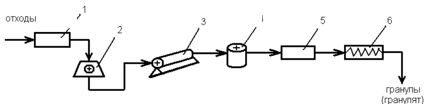
Рис. 1.1. Схема вторичной переработки полиолефинов в гранулы: 1 – узел сортировки отходов; 2 – дробилка; 3 – моечная машина; 4 – центрифуга; 5 – сушильная установка; 6 – гранулятор
