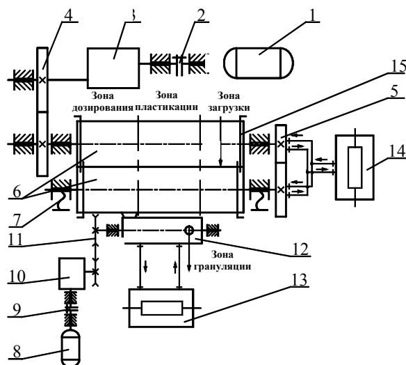
Рис. 2.2. Схема лабораторной установки:
