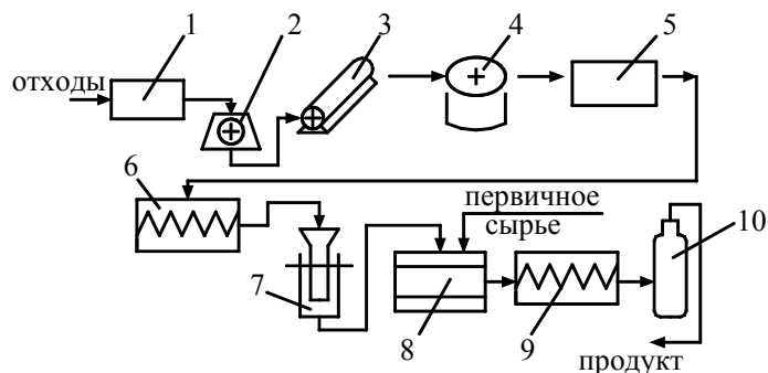
Рис. 2.5. Схема производства вторичной ПЭ тары
