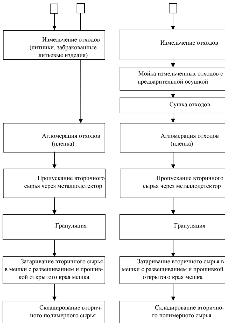
Рис. 2.4. Продолжение
