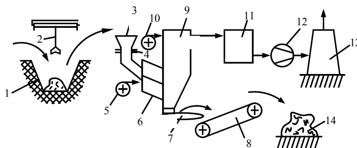
Рис. 2.7. Схема установки термического обезвреживания твердых полимерных отходов
